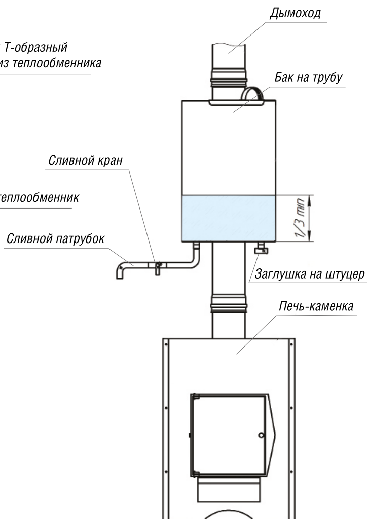
СХЕМА МОНТАЖА БАКА ДЛЯ ПЕЧИ С ТРУБОЙ
